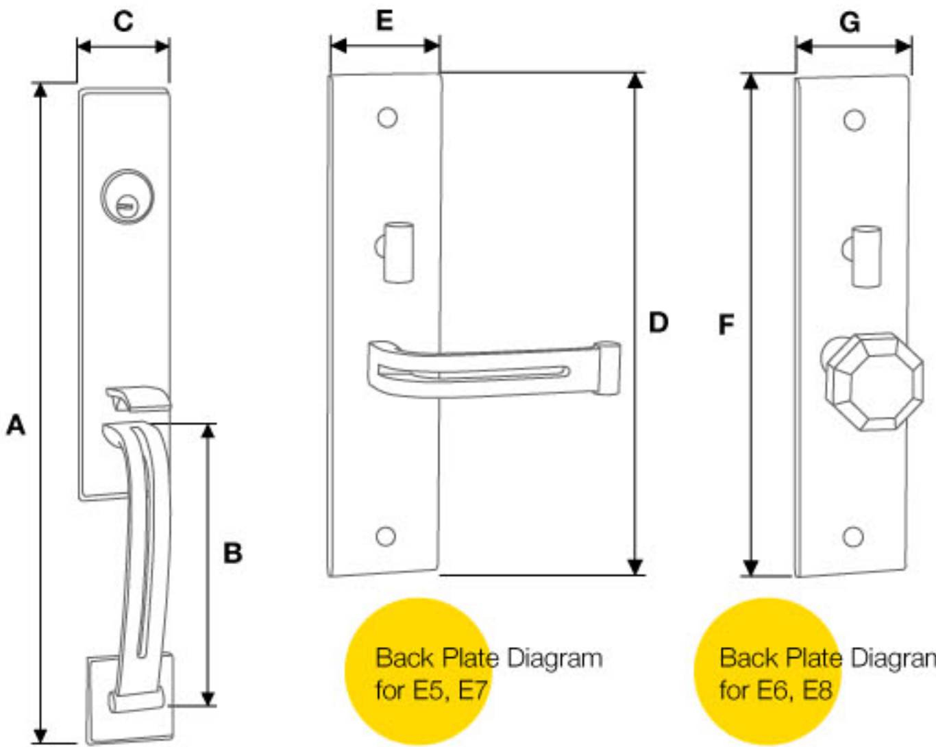
Front Plate Diagram for E5, E6, E7, E8
